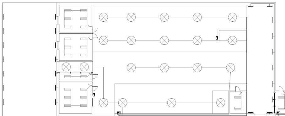
Plano con instalación eléctrica de luminaria.
